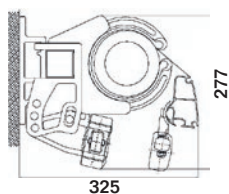
Instalación en la pared (en mm.)
