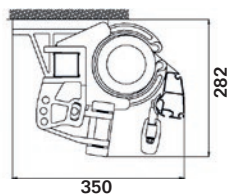
Instalación en el techo (en mm.)
